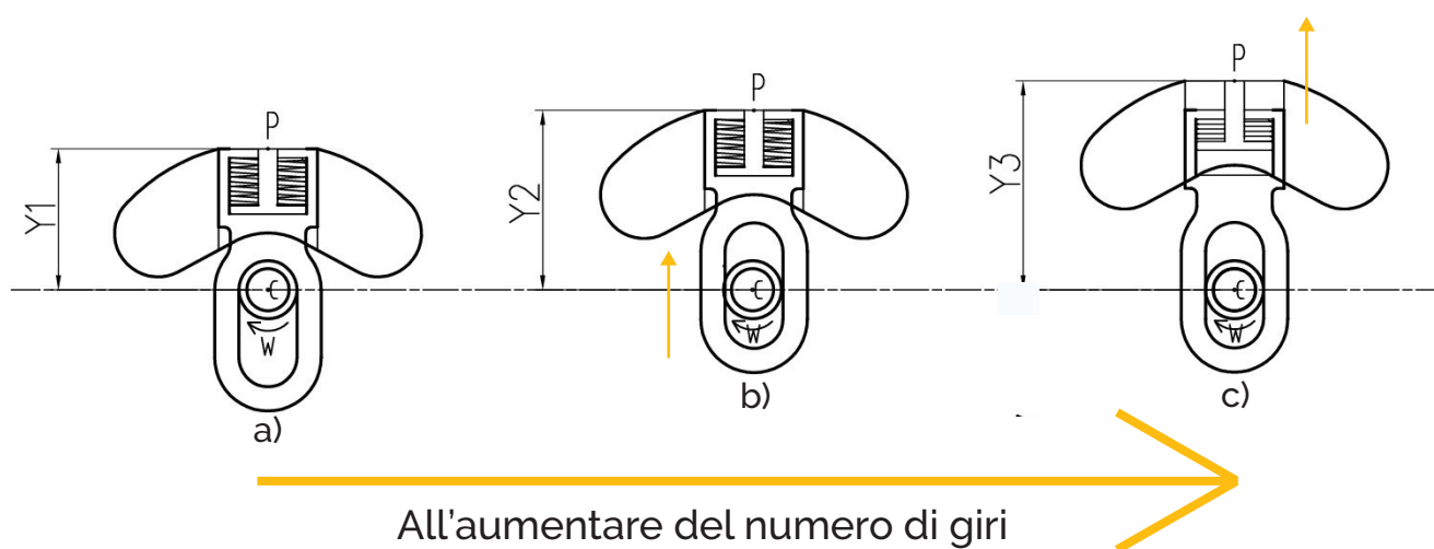
Fig. 3: variazione spaziale delle masse eccentriche all'aumentare del numero di giri
