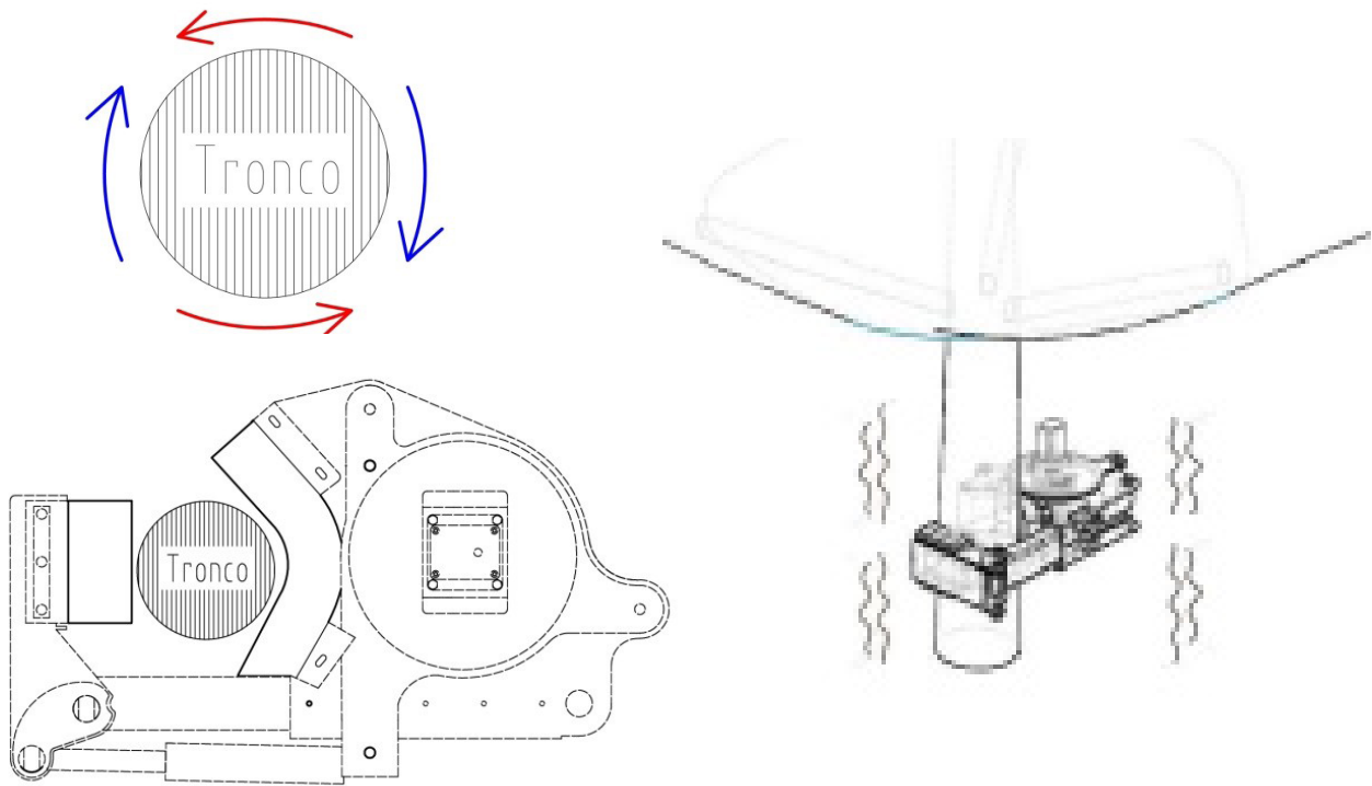
Fig. 4: all'atto della vibrazione, il tronco presenta sollecitazioni torsionali minime (freccie in rosso e blu)
