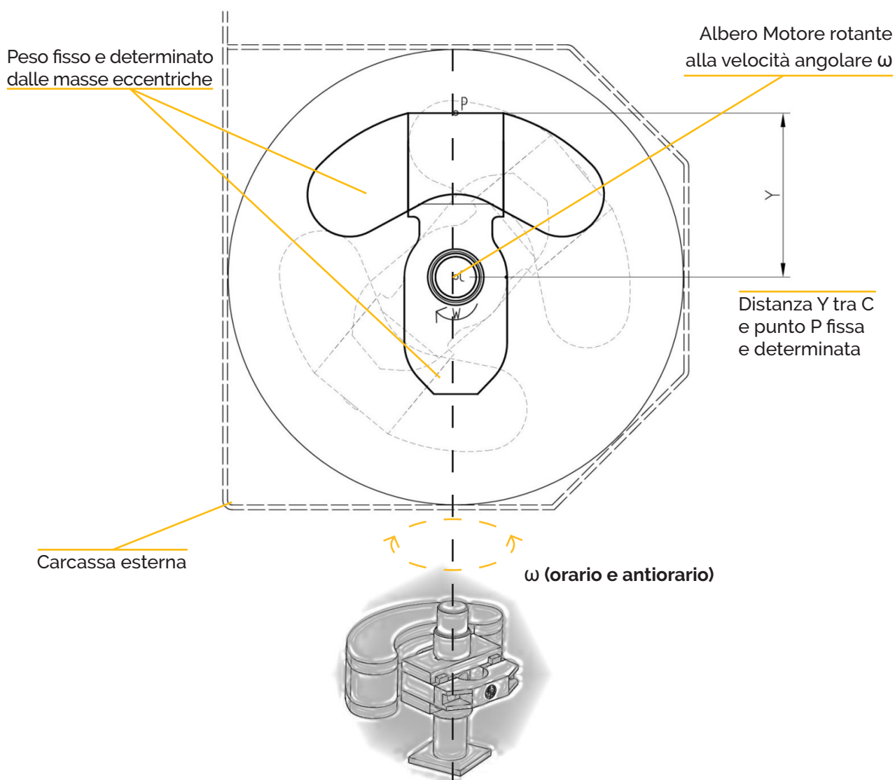
Fig. 1: masse eccentriche nei comuni scuotitori sul mercato
