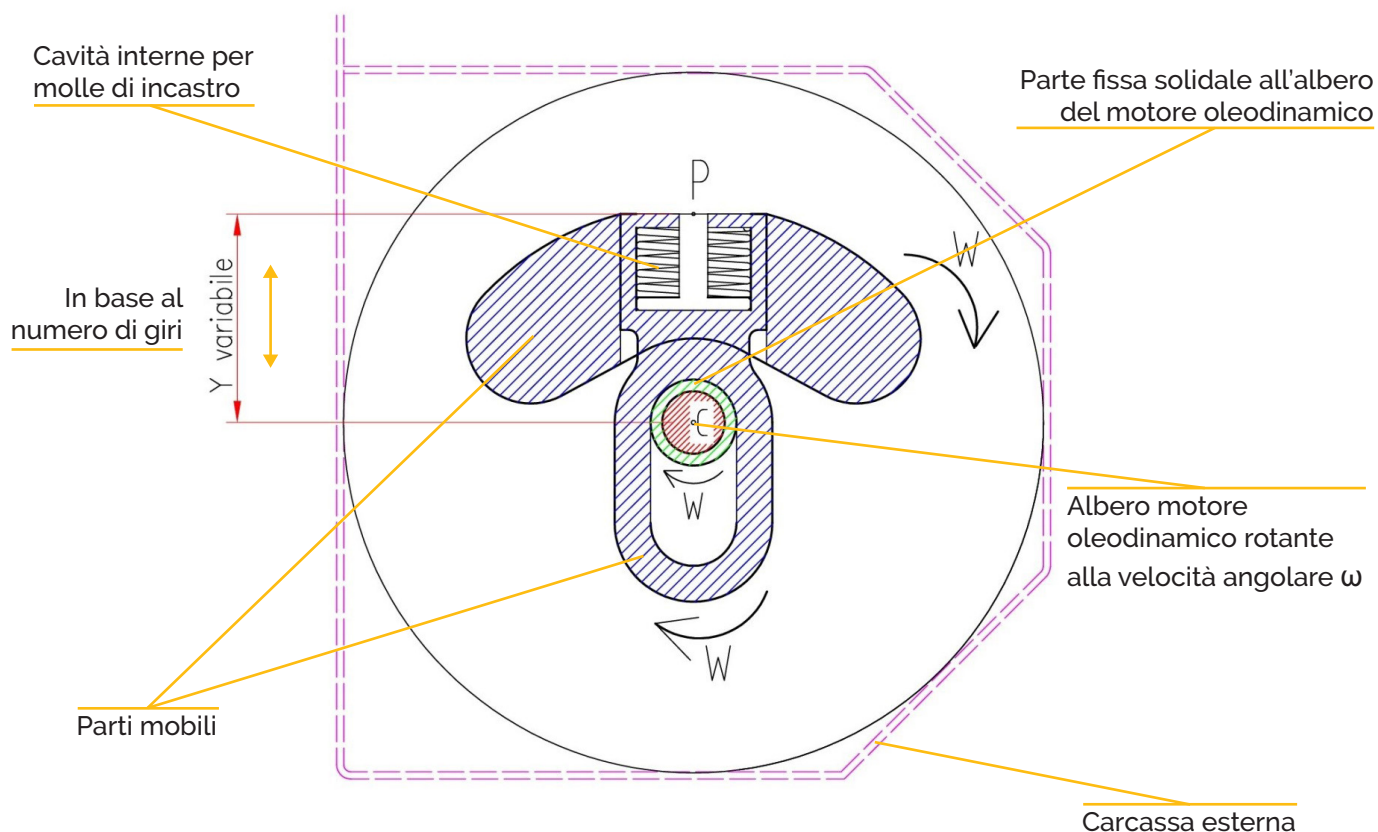
Fig. 2: masse eccentriche scuotitori S.P.A.R.E.
